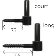
Gond à visser
