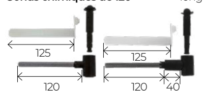
Gonds chimiques de 120
