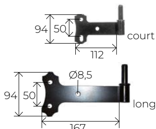
Gond à plaquer
