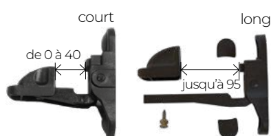
Gond sur platine
