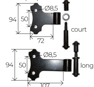
Gond à plaquer
