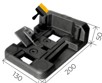
Sabot avec basculeur en cupro-aluminium
