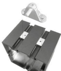
Contre plaque alu pour gond inox pour poteau 180 uniquement
