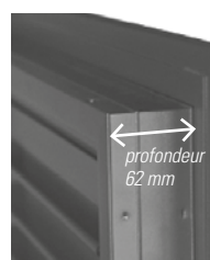
Précadre côté intérieur
