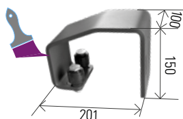
Guidage haut en aluminium pour portails forme droite
