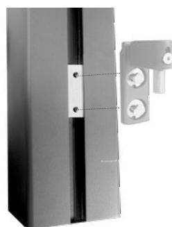
Contre plaque alu pour gond multiréglable
