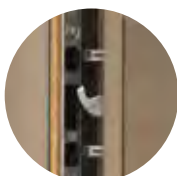
Point de fermeture hauts : - 2 goujons - 1 crochet
