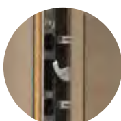
Point de fermeture bas : - 2 goujons - 1 crochet
