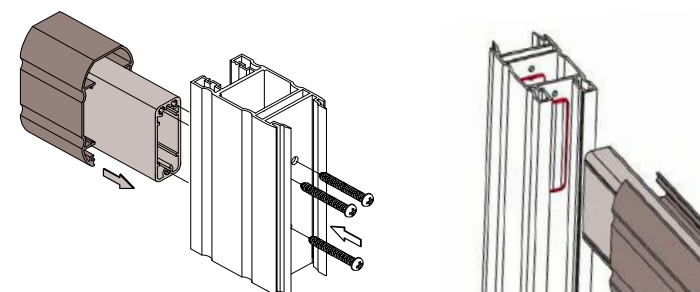
Exemple tenon-mortaise double.
