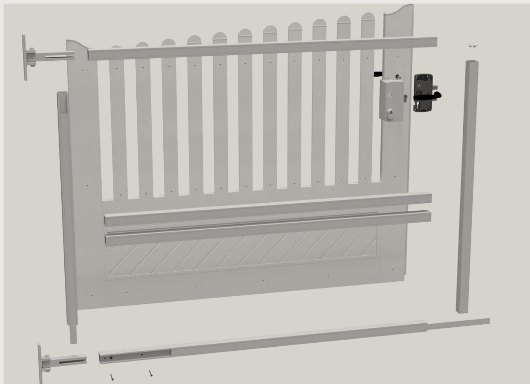
Eclaté vue de derrière
